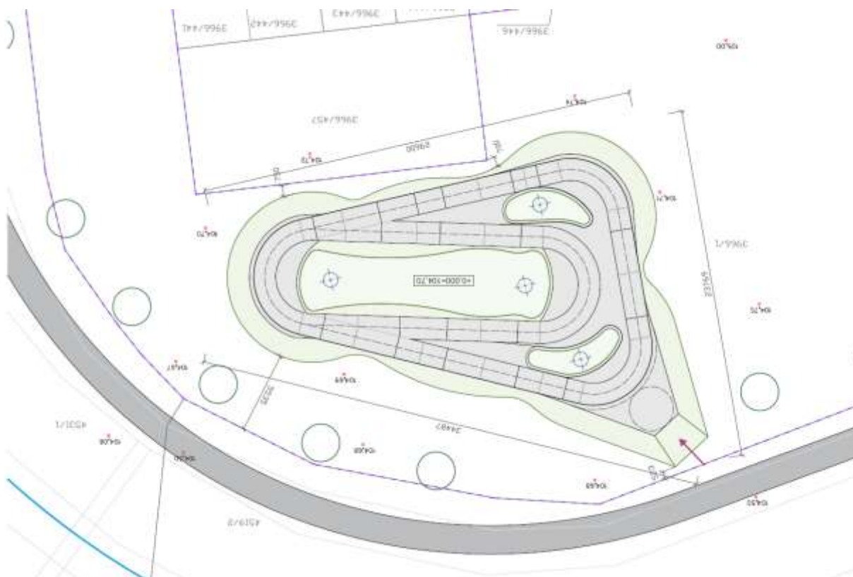
Navrhovaná stavba
